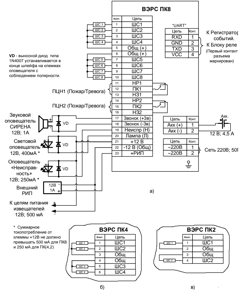
Рис.2. Схемы внешних соединений приборов ВЭРС-ПК(8,4,2)(П,М) версия 2
